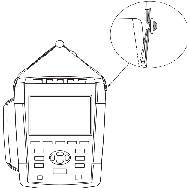
图 4-2. 固定挂带
