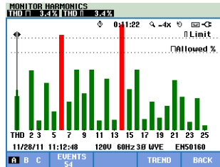
图 16-4. 条形图屏幕
