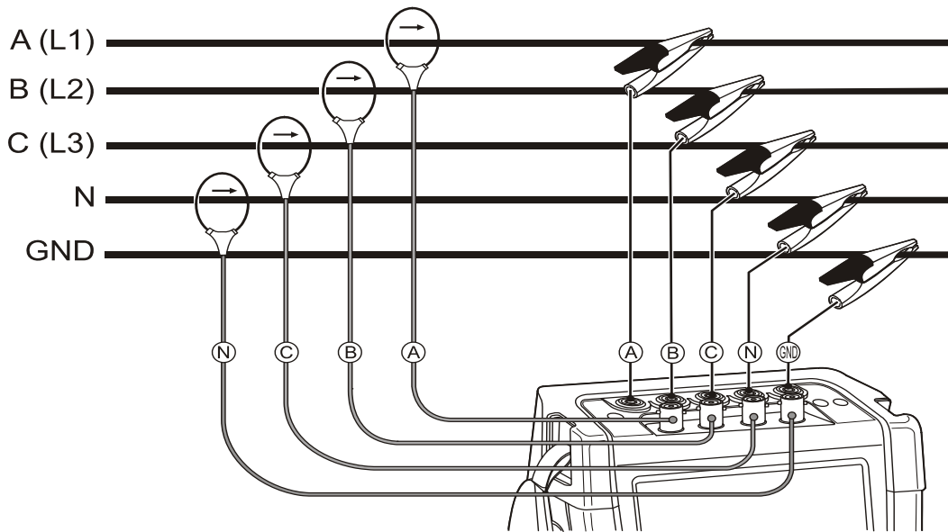
图 6-2. 将分析仪与三相配电系统连接
