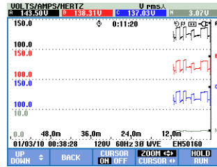
图 23-6. 趋势图显示（光标和缩放功能启用）
