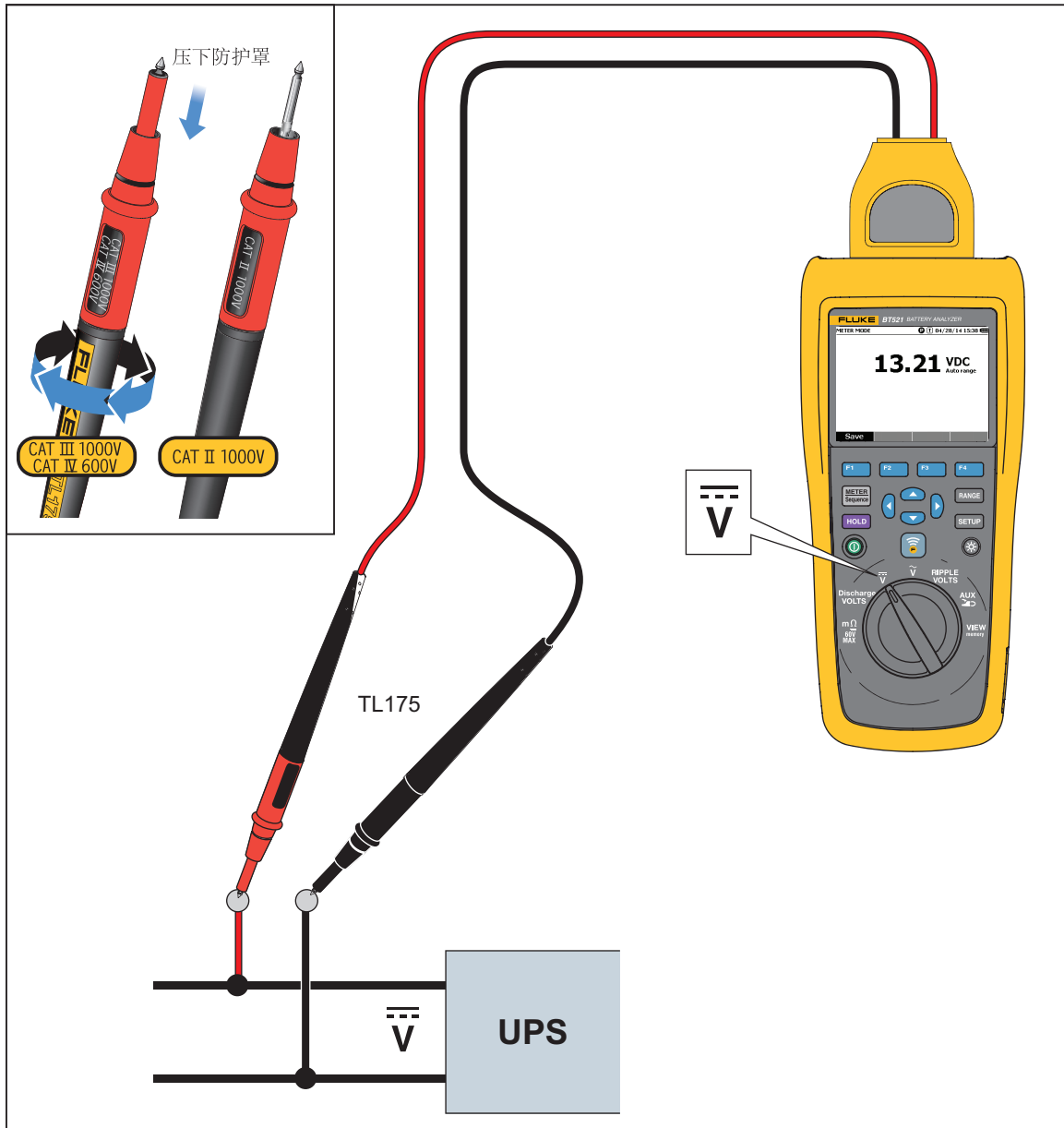
图 3-6. 测量直流电压
