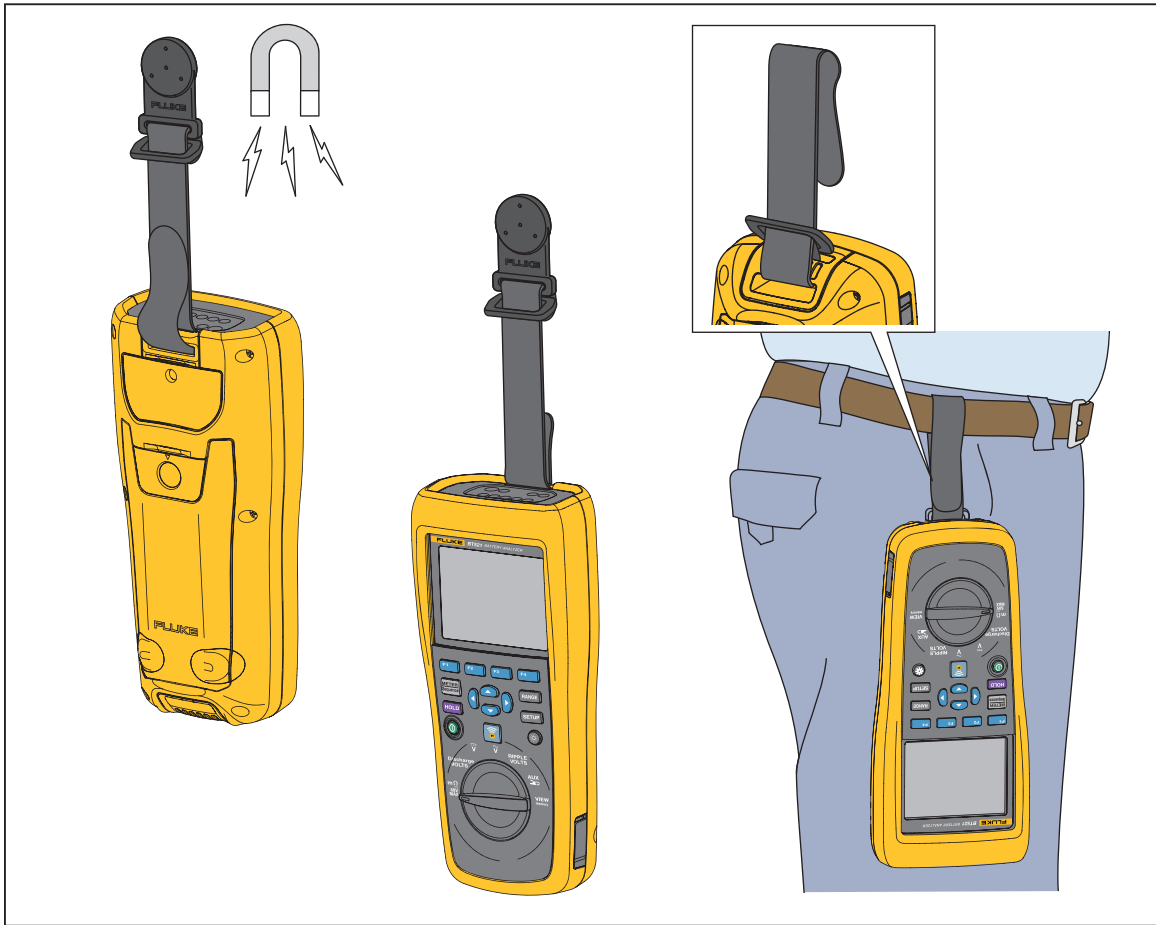
图 2-2. 挂带
