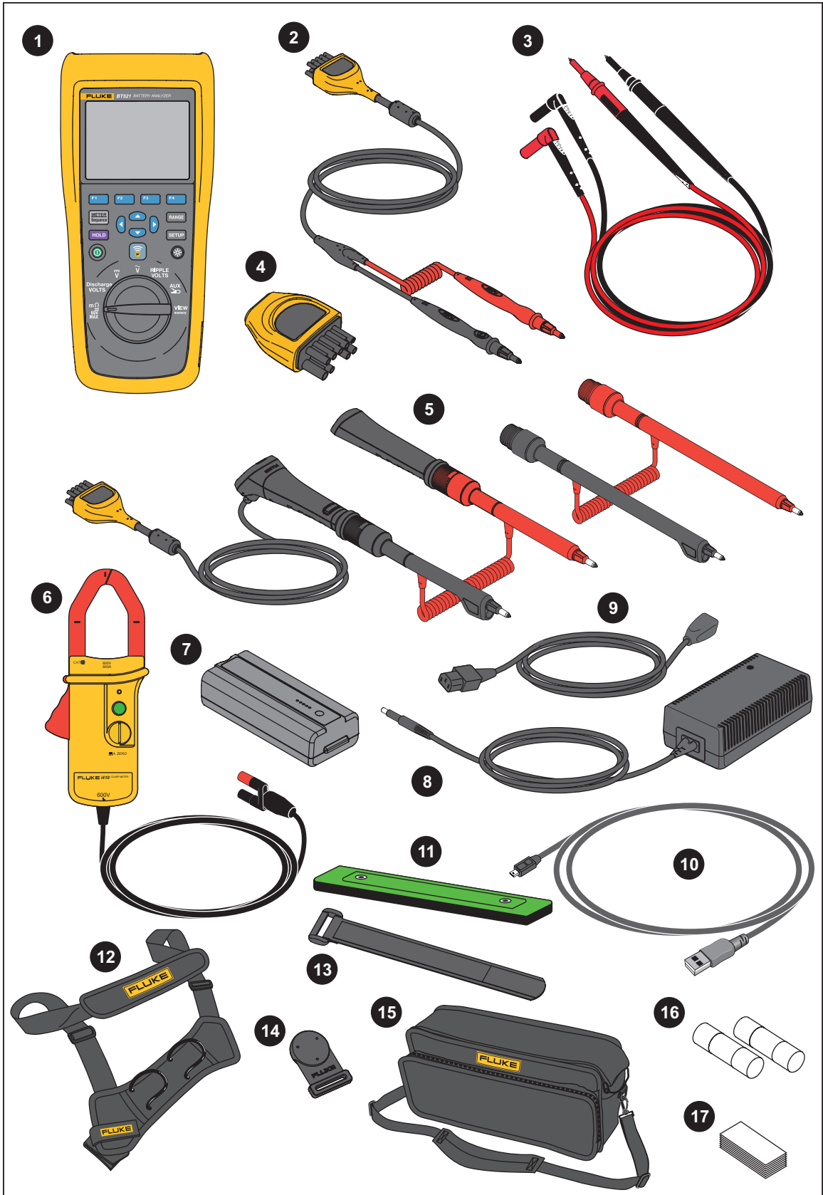
图 1-1. 标准设备
