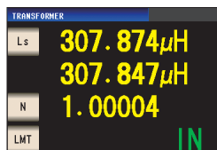
变压器测量模式 卷数比测量·判断界面
