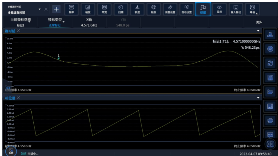
多载波群延时测量界面
