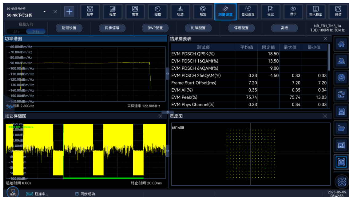
5G NR 信号分析界面
